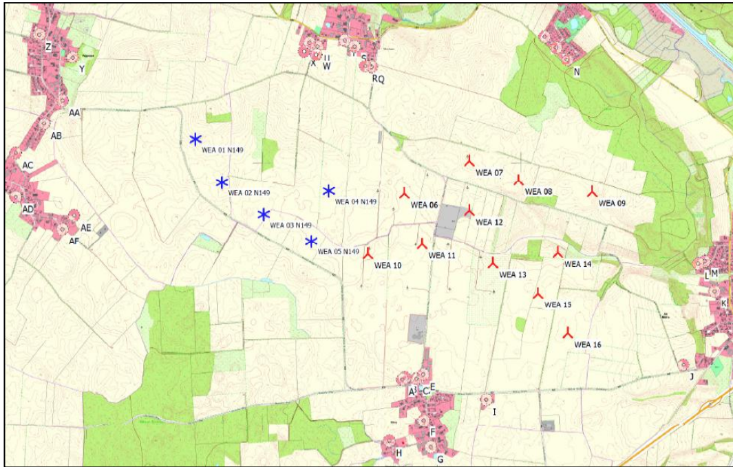
Abb. 8: Immissionspunkte (IP) und Schallquellen (Vorbelastung und Zusatzbelastung) als Gesamtbelastung im Vorranggebiet PR3_LAU_033 (verändert nach PLANKon 2025a)
